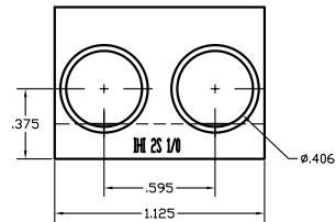
IHI 2S1/0, WIRE RANGE 1/0-14
