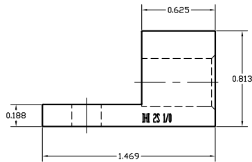
IHI 2S1/0, WIRE RANGE 1/0-14
